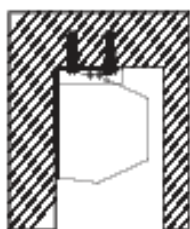
Встроенная установка на расширительные болты
