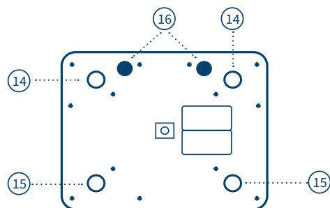
Вид нижней панели проектора
